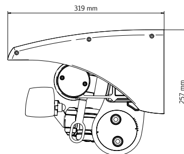
Sprängskiss med tak
