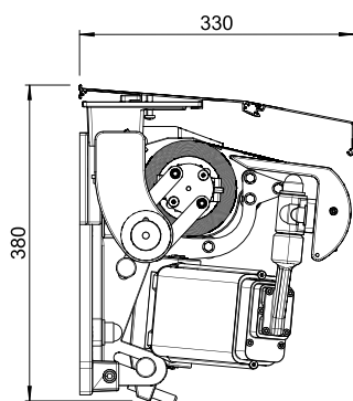
Väggmonterad TM8900 med skyddstak
